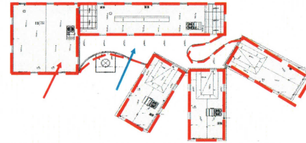
Planta de Conjunto nivel 1-125 Adecuación y Mejoras de la Cubierta y "Huerto Solar" en la Biblioteca Central del Campus Norte.
