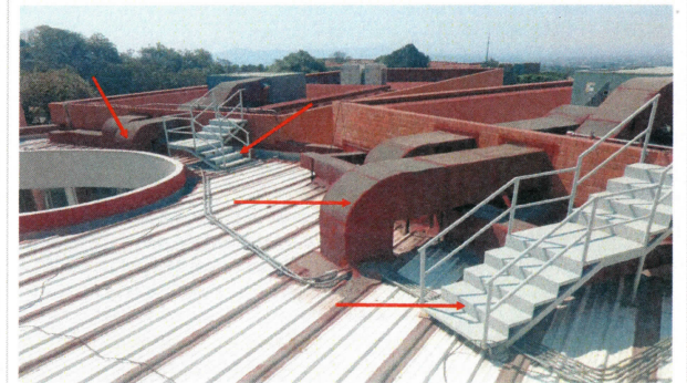
F5: Adecuación y Mejoras de la Cubierta y "Huerto Solar" en la Biblioteca Central. Retiro de ductos de aire acondicionado, escaleras metálicas y sustitución de cubierta.
