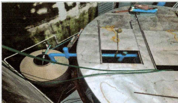
Trabajos de, suministro, instalación, pruebas y puesta en funcionamiento de tuberías y accesorios, en la Facultad de Contaduría, Administración e Informática.
