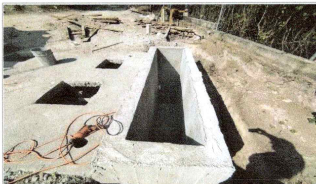
Instalación, prueba y puesta en funcionamiento de tablero del sistema de clorador, con canal desnatador y clorador, Escuela de Estudios Superiores del Jicarero.
