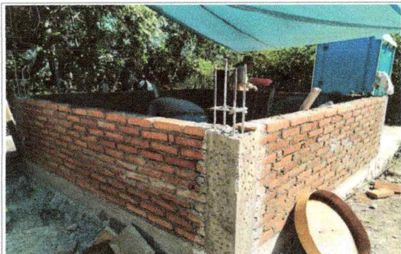
Trabajos de suministro e instalación, conexión y pruebas de tolva para secado de lodos en la Escuela de Estudios Superiores del Jicarero.
