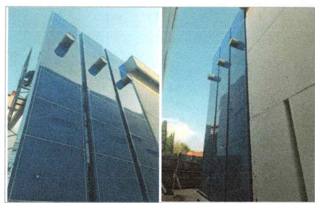
Trabajos de suministro y colocación de panel compuesto de aluminio (ALUCUBOND) en el Centro de Investigaciones Químicas (CIQ).
