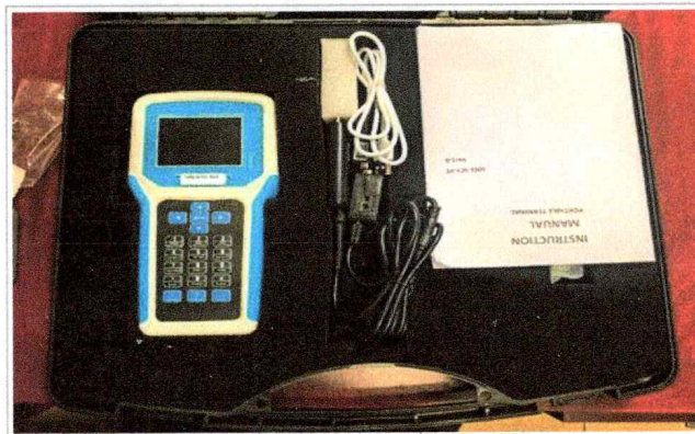
Probador de suelos 7 en 1 con terminal de pantalla LCD portátil marca QT Escuela de Estudios Superiores de Xalostoc
