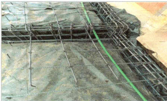
Trabajos de suministro y tendido de instalación hidráulica, en la Facultad de Ciencias Químicas e Ingeniería (TAMULBA).
