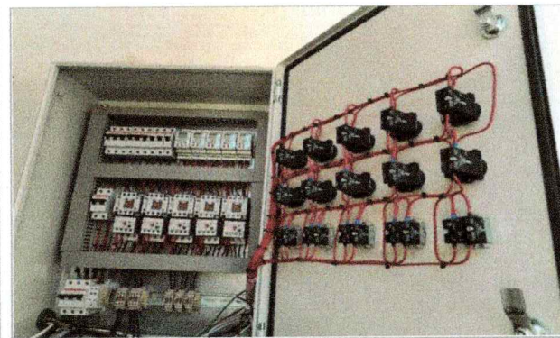
Trabajos de tablero de control e interruptores, Escuela de Estudios Superiores del Jicarero.
