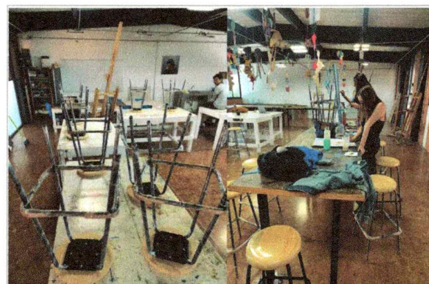
Bancos de laboratorio fabricados en estructura tubular redondo de \frac{1}{2} calibre 18 para el Taller de pintura 2 de la Facultad de Artes
