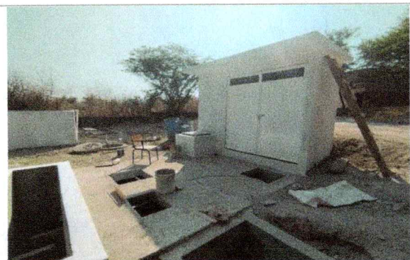
Trabajos de cobertizo para resguardo de equipos, Escuela de Estudios Superiores del Jicarero.
