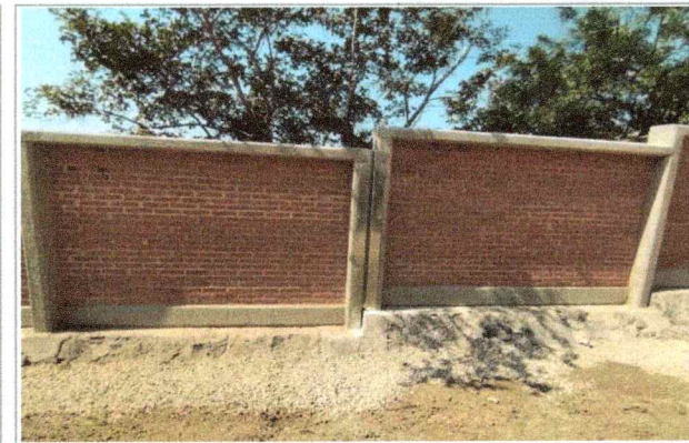
Trabajos de suministro e instalacion, tapa junta con lámina galvanizada, en la Escuela de Estudios Superiores de Atlaltlahucan.
