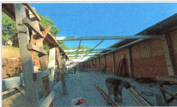
Trabajos de estructura metálica (acero misceláneo/ placas, cartabones, anclas, pernos), en la Facultad de Ciencias Químicas e Ingeniería (TAMULBA).
