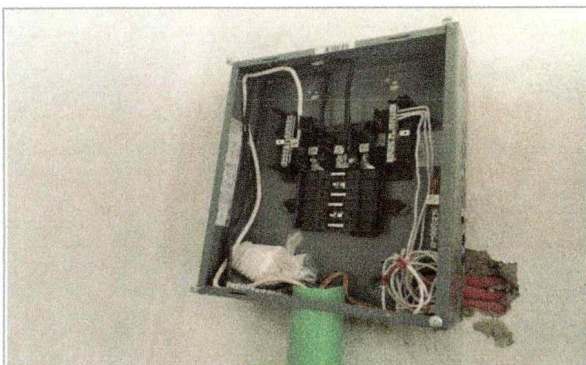
Trabajos de suministro e instalación de centro de carga, Escuela de Estudios Superiores del Jicarero.
