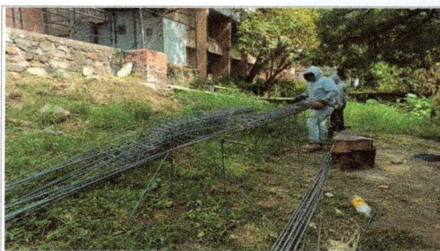
Trabajos de habilitado de acero de refuerzo en la Facultad de Ciencias Químicas e Ingeniería (TAMULBA).
