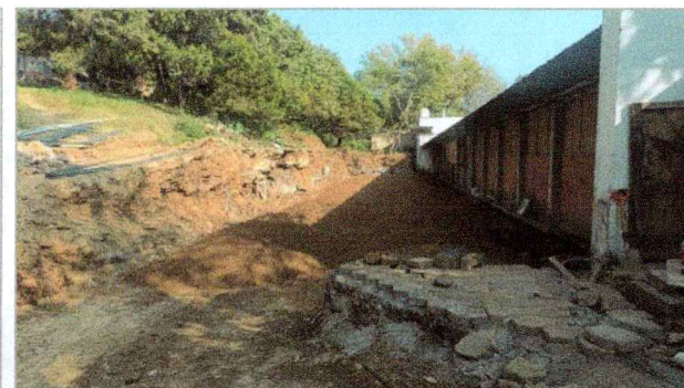
Trabajos de tendido de relleno de material de banco tepetate compactado por medios mecánicos, en la Facultad de Ciencias Químicas e Ingeniería (TAMULBA).
