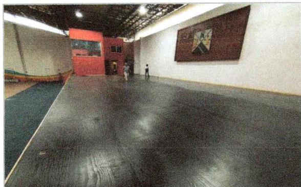
Trabajos de piso flotado de triplay y banda de neopreno en el perímetro, para el edificio A-20 Gimnasio Auditorio.
