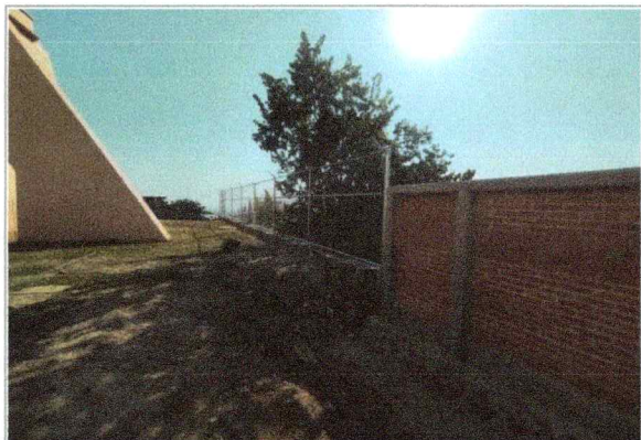
Trabajos de suministro e instalacion de malla ciclonica galvanizada, en la Escuela de Estudios Superiores de Atlaltlahucan.
