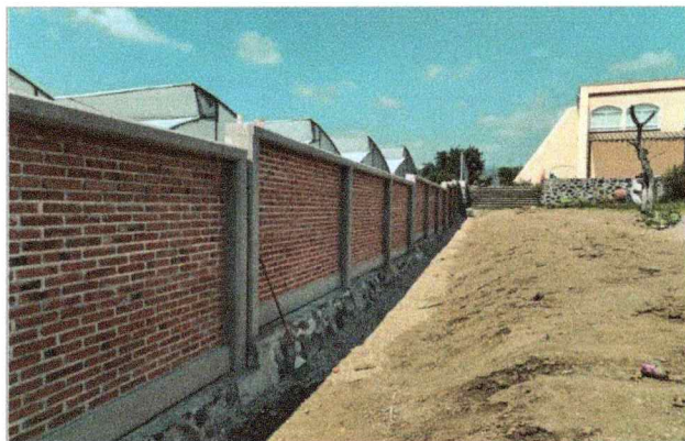
Trabajos de filtro de grava triturada, así como la colocación de dren de PVC 4", en la Escuela de Estudios Superiores de Atlaltlahucan.
