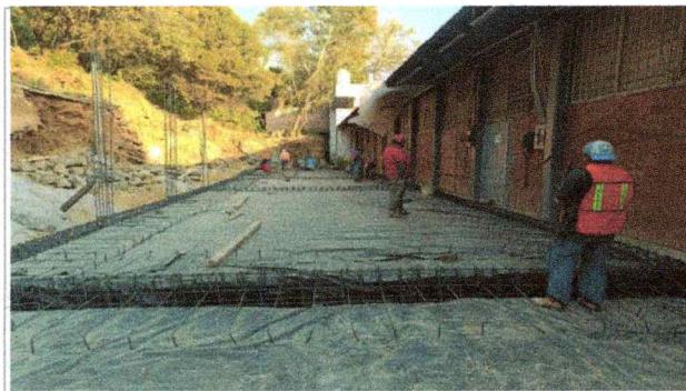
Trabajos de suministro y colocación de membrana de polietileno en la Facultad de Ciencias Químicas e Ingeniería (TAMULBA).
