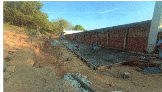
Trabajos de firme de concreto reforzado con malla electrosoldada, en la Facultad de Ciencias Químicas e Ingeniería (TAMULBA).
