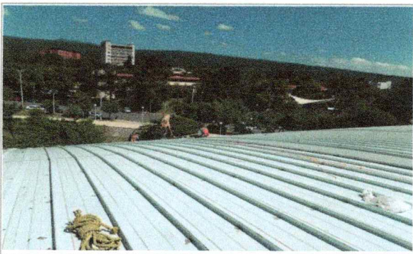
Trabajos de reparación de sellos en cubierta existente, en el edificio A-37 Polideportivo 01.
