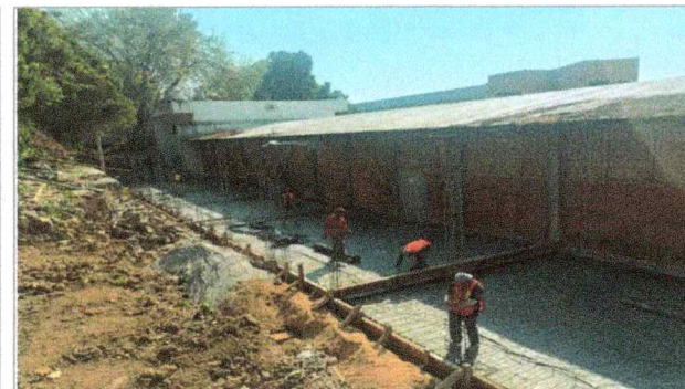
Trabajos de acero de refuerzo (cadenas, castillos y anclas), en la Facultad de Ciencias Químicas e Ingeniería (TAMULBA).
