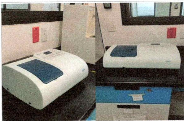
Espectrofotómetro UV Vis, Rango de longitud de onda: 190-1100 nm; Ancho de banda espectral: 2 nm; Precisión de longitud de onda: \pm 0.8 . Repetibilidad de la longitud de onda: 0.3 nm. Calibración de longitud de onda automática. Deslizador con 4 celdas estándar de 10 mm para el Laboratorio - Planta Piloto (Edificio 61) en la Facultad de Farmacia.
