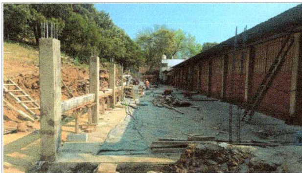
Trabajos de cimbrado y colado de concreto de cadenas y castillos en la Facultad de Ciencias Químicas e Ingeniería (TAMULBA).
