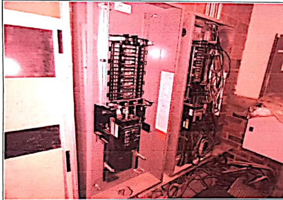
F1: Tableros eléctricos actuales
