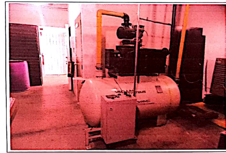
F5: Bomba General de vacío
