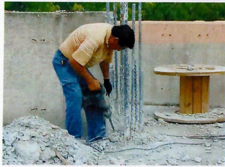
F7: Demolición de concreto que recubría al acero de columnas.
